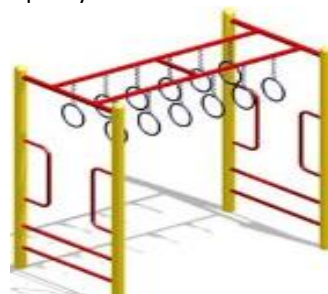
Гимнастический комплекс 2300*700*2500мм
